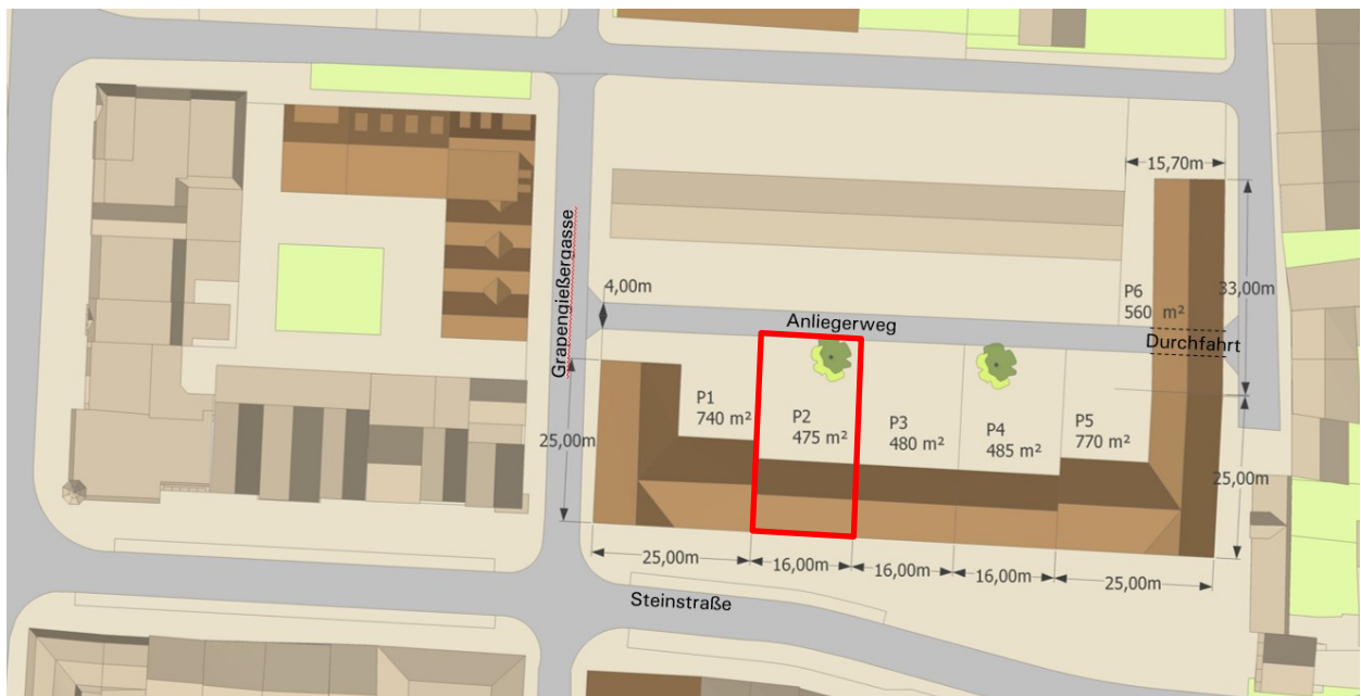
Abb. Parzellierungsvorschlag
